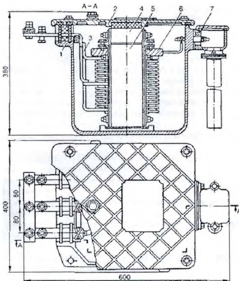
Рис. 1. Основные узлы дроссель-трансформатора ДТ-0,2-500
