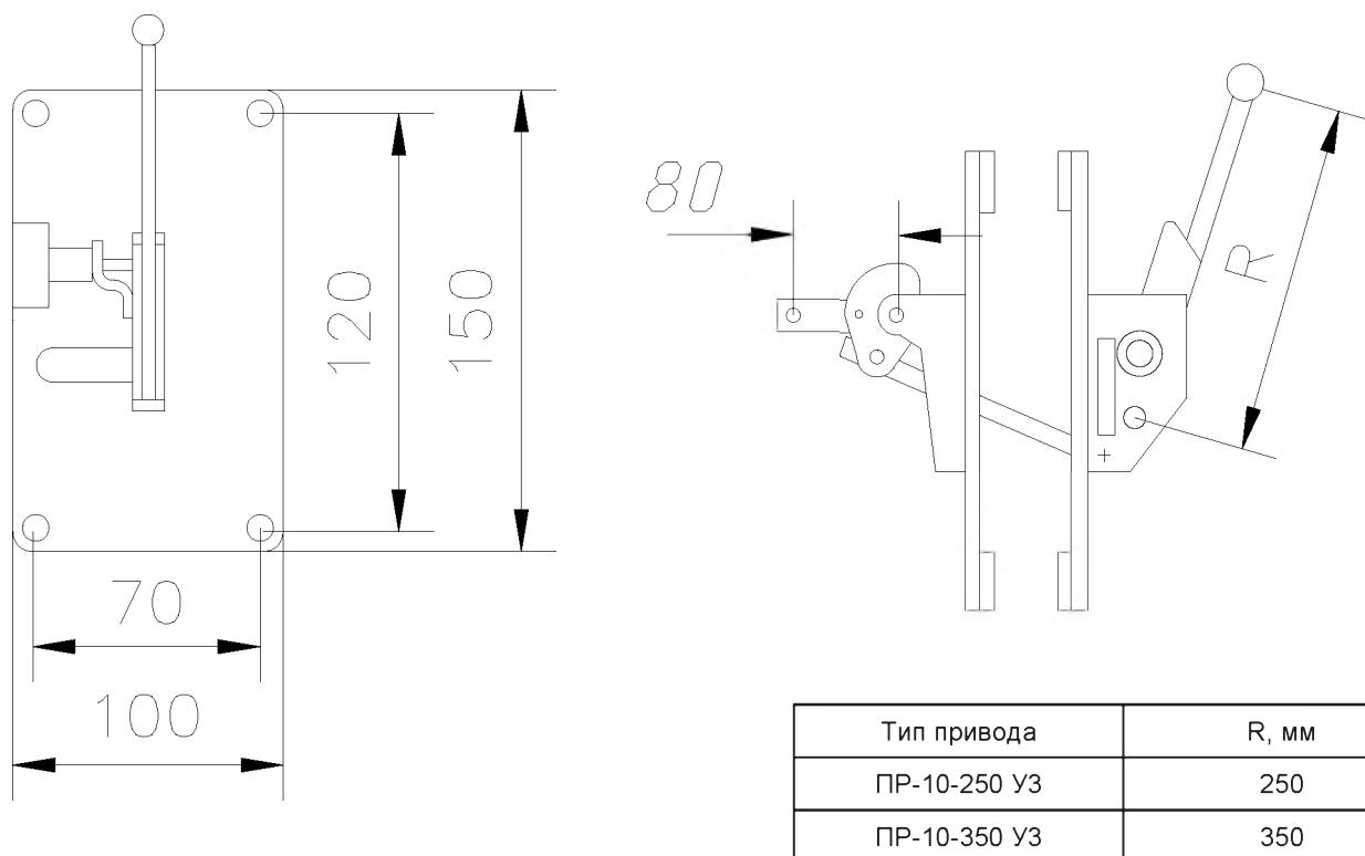
Рисунок 2. Общий вид, габаритные и установочные размеры привода ПР-10
